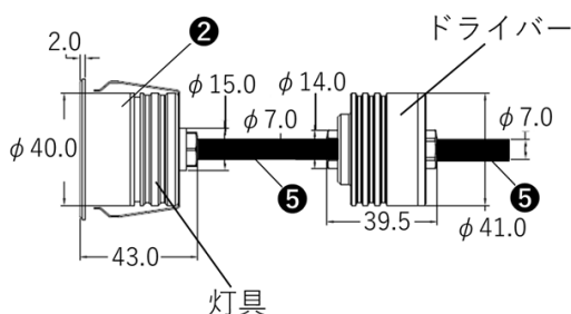
(灯具横断面寸法)
