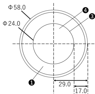
(灯具上面寸法)
