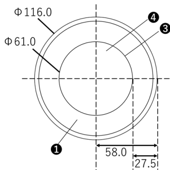
(灯具上面寸法)
