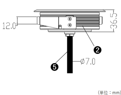
(灯具横面寸法)
