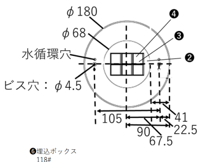
(灯具上面寸法)
