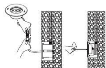
6. 本体の電源ケーブルと枠のケーブルをつなぎ、本体を枠にネジで固定します。
