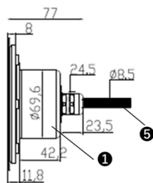
(灯具横面寸法)
