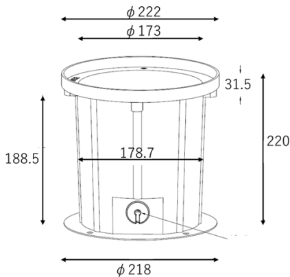
(横面寸法)
