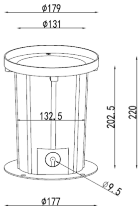
(横面寸法)
