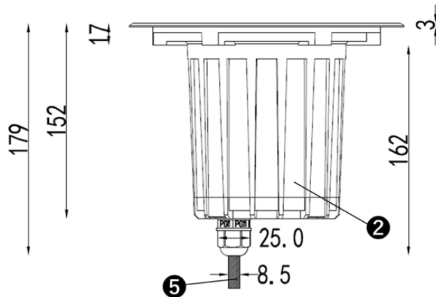
(灯具横面寸法)
