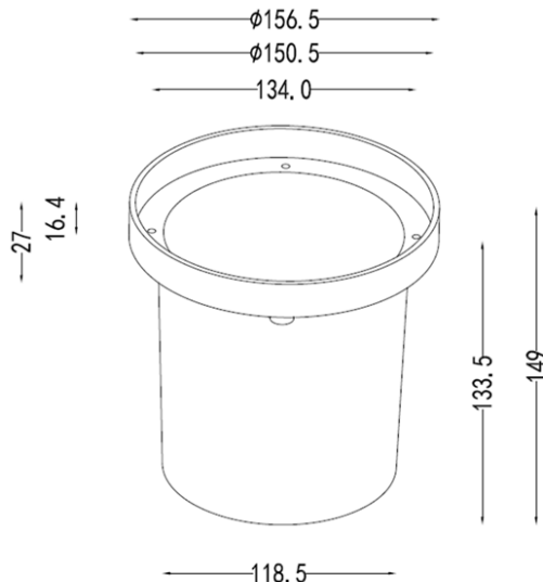
(横断面寸法)
