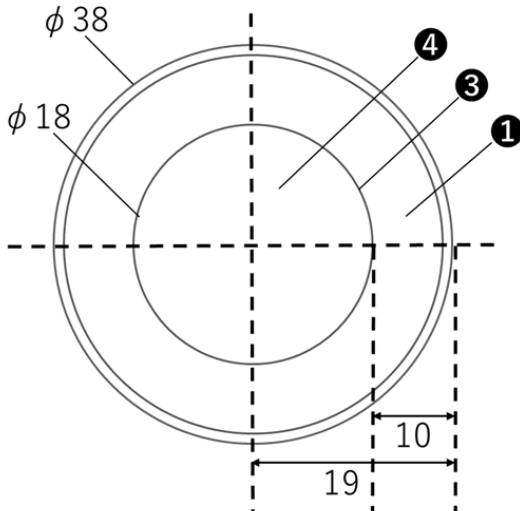
(灯具上面寸法)
