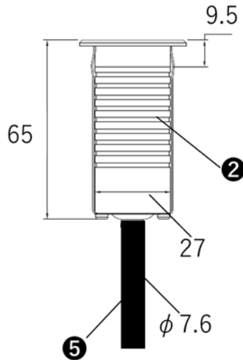
(灯具横断面寸法)
