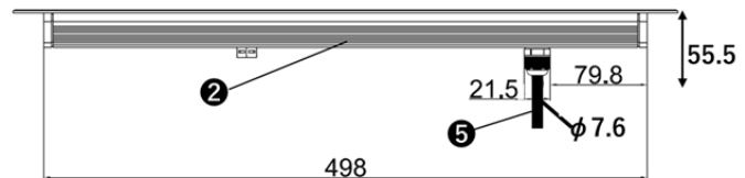
(灯具横面寸法)
