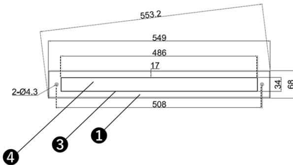
(灯具上面寸法)
