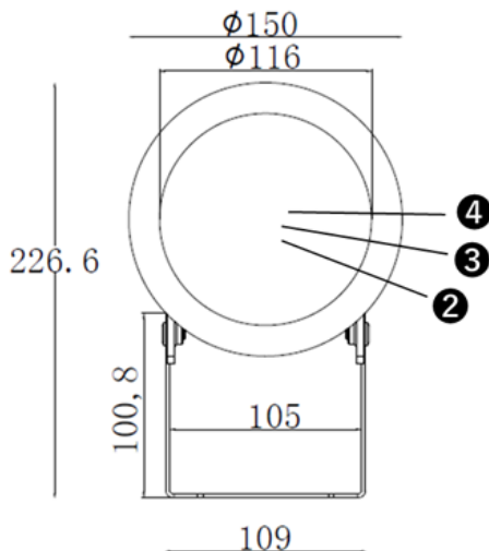
(灯具正面寸法)
