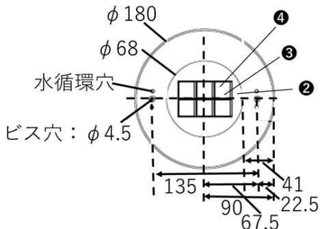
(灯具上面寸法)
