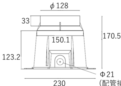
(横断面寸法)
