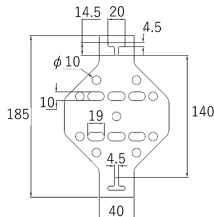
(取付金具寸法)
