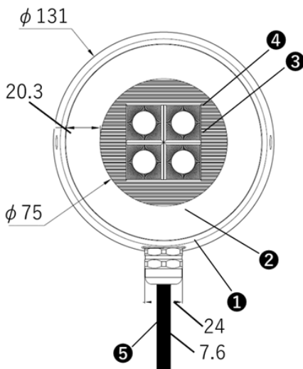
(灯具上面寸法)
