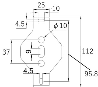
(取付金具寸法)
