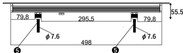
(灯具横断面寸法)
