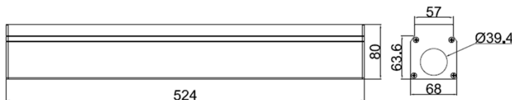
(横断面寸法)
