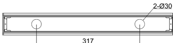
(上面寸法)
