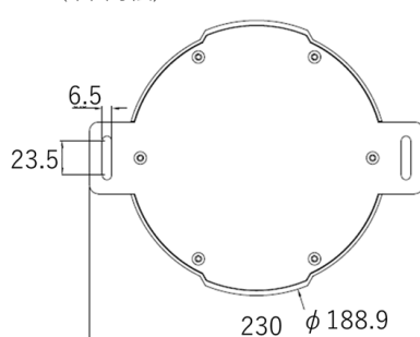
(下面寸法)
