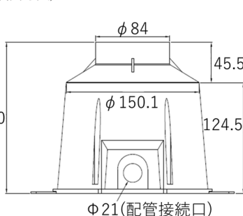
(横断面寸法)
