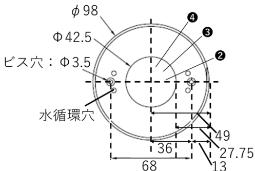
(灯具上面寸法)
