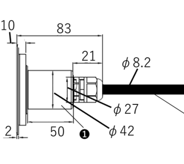
(灯具横断面寸法)
