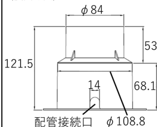
(横断面寸法)
