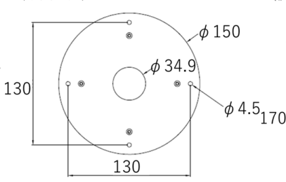
(下面寸法)
