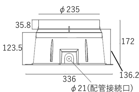
(横断面寸法)
