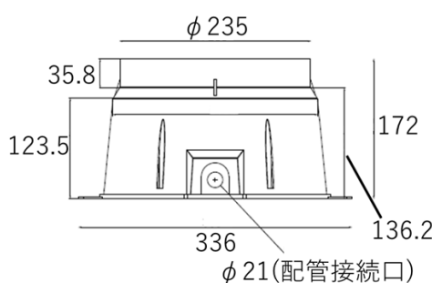
(横断面寸法)
