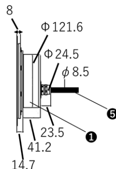
(灯具横断面寸法)
