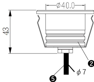
(灯具横断面寸法)
