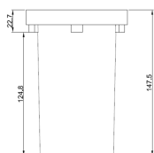
●埋込ボックス 015#(標準) (横面寸法)
