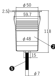
(灯具横面寸法)
