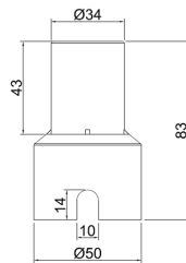
(横面寸法)
