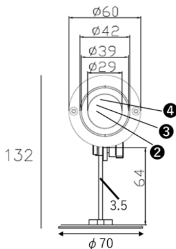
(灯具正面寸法)
