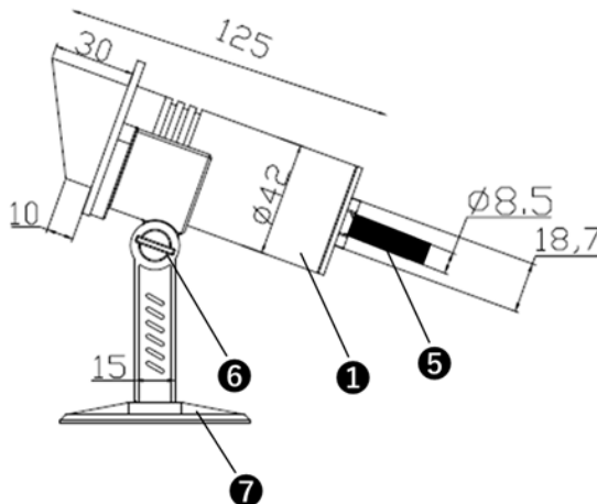
(灯具横断面寸法)
