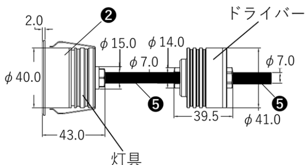
(灯具横面寸法)
