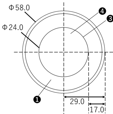
(灯具横面寸法)
