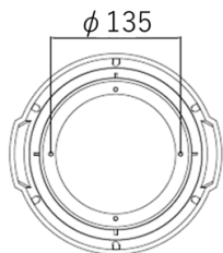
(上面寸法)
