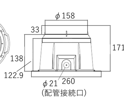
(横断面寸法)
