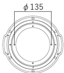
(上面寸法)
