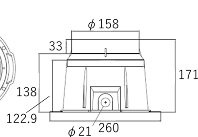
(配管接続口)
