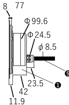
(灯具横断面寸法)
