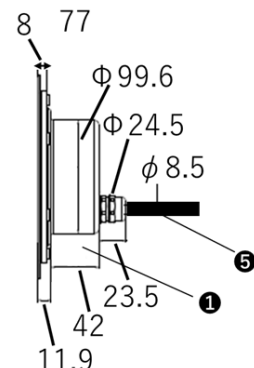
(灯具横断面寸法)
