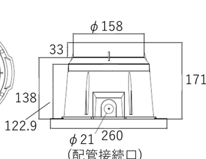
(横断面寸法)
