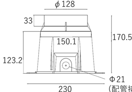
(横面寸法)
