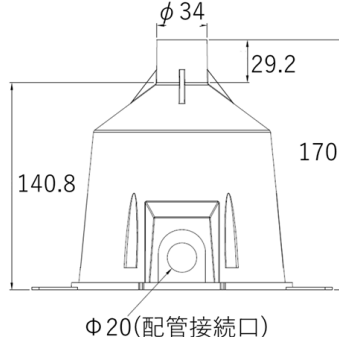
(横断面寸法)
