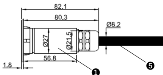
(灯具横断面寸法)
