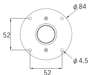
(下面寸法)
