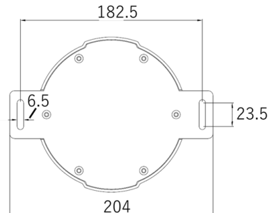
(下面寸法)
