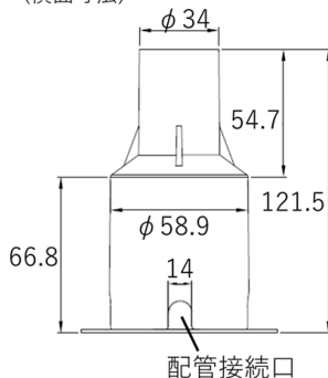
(横断面寸法)
