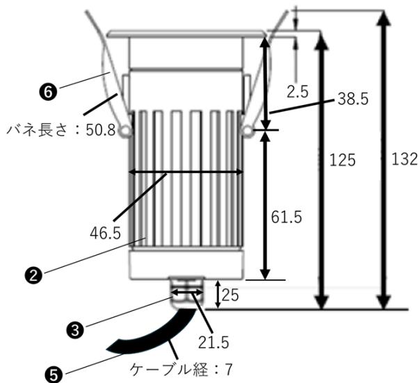
(灯具横断面寸法)
