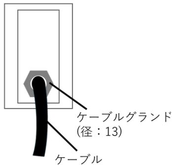
ケーブル
