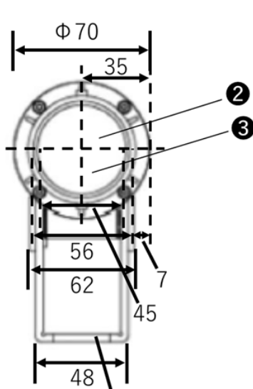
台座の厚み：5
