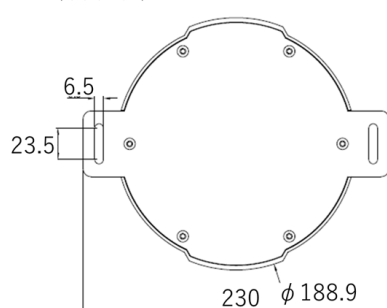
(下面寸法)
