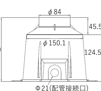
(横断面寸法)
