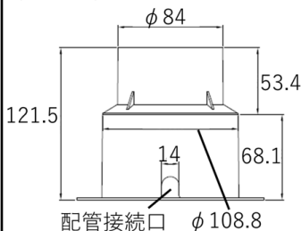
(横断面寸法)
